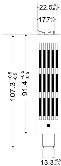
俯视图
