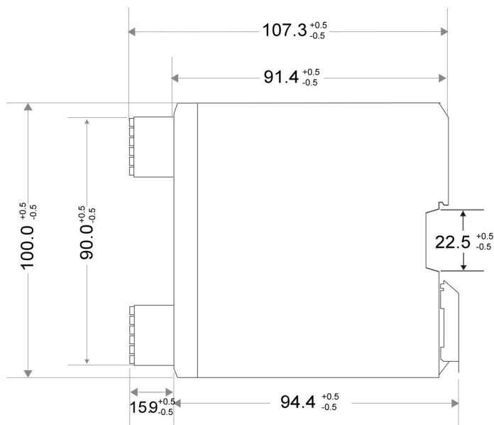
侧视图
